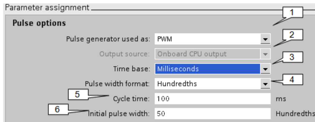
图4 脉冲发生器组态
