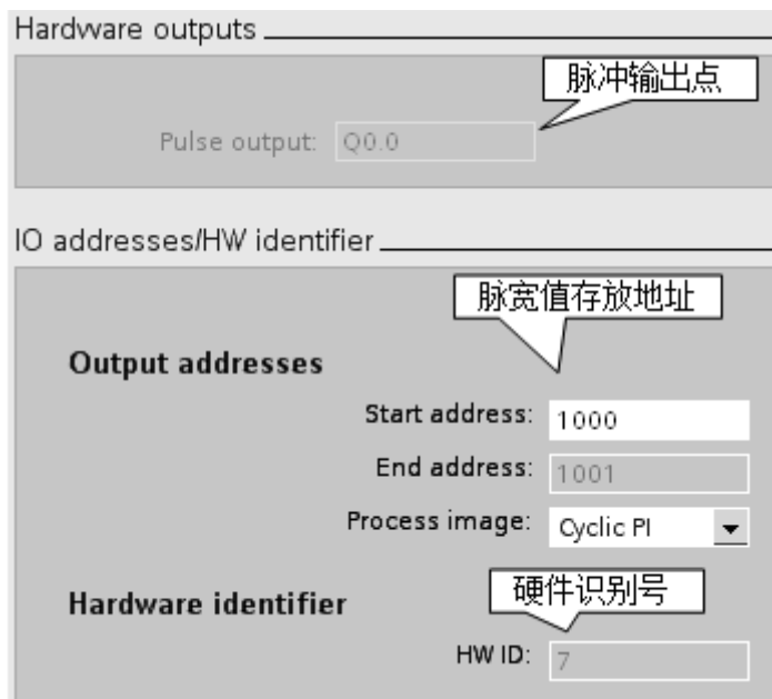
图9 硬件输出点与脉宽地址
